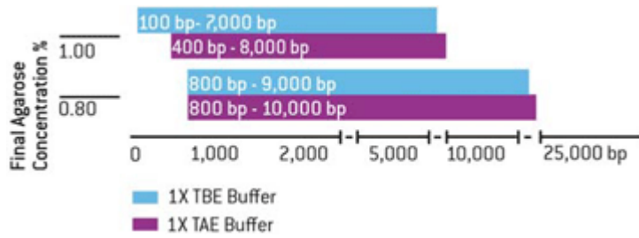
Abb. Trennverhalten SeaKem LE
