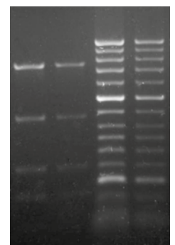
Auftrennung verschiedener Marker (bis 2 kb) in 1%iger Biozym LE Agarose, TBE Puffer, In-Gel Färbung, Midori Green Advance
