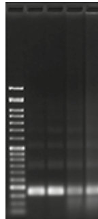
168 bp Ampikon, erzeugt mit biotechrabbits RPA Basic Master Mix, dargestellt in einem Agarosegel.
